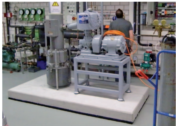
Vollflächige Maschinenfundamentlagerung mit Regupol®
