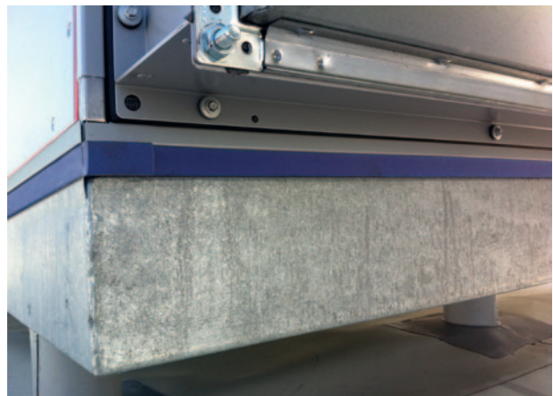
Samson Produktionsgebäude, Offenbach am Main: Streifenförmige Schwingungsisolierung klimatechnischer Anlagen
