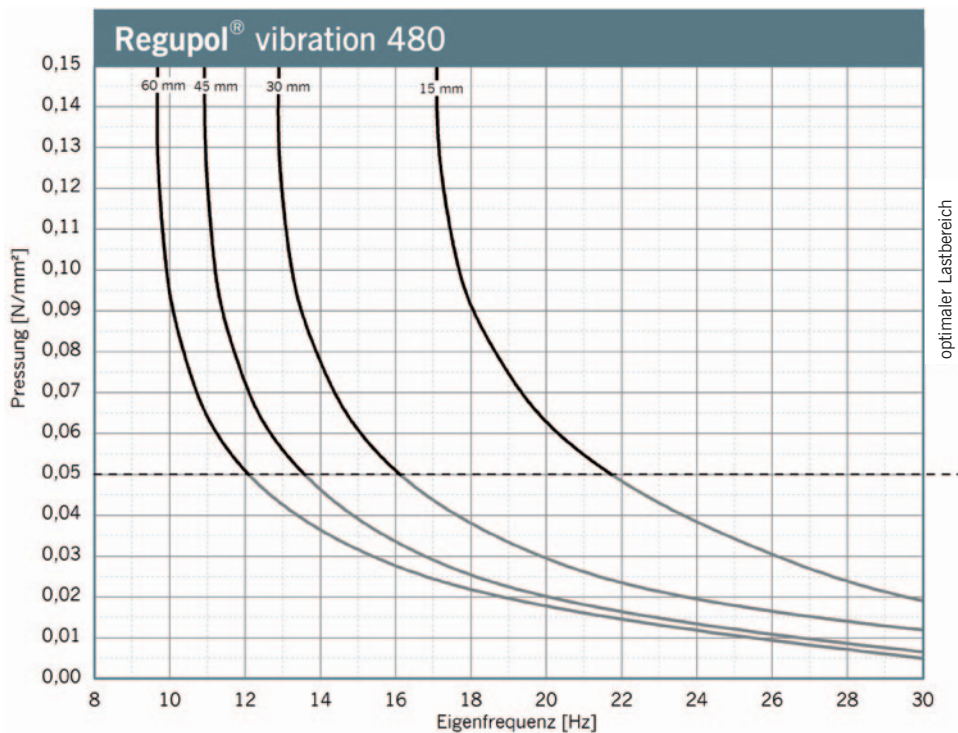
Eigenfrequenzverläufe für einen eindimensionalen Feder-Masse-Schwinger unter Berücksichtigung der dynamischen Steifigkeit von Regupol® vibration 480 auf starrem Untergrund. Probenabmessung 300 mm x 300 mm.
