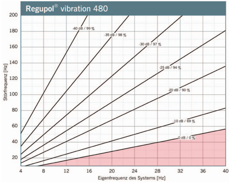
Dargestellt ist die Isolierung für einen Ein-Massen-Schwinger auf starrem Untergrund mit Regupol® vibration 480 . Parameter: Kraftübertragungsmaß in dB, Isolierwirkungsgrad in %.
