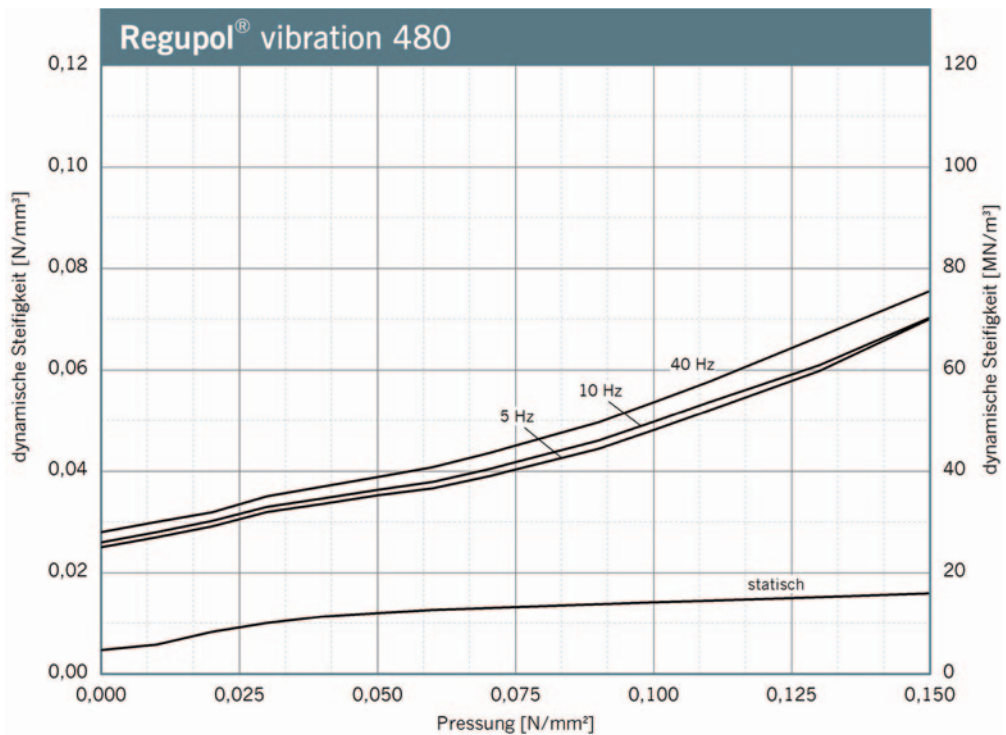
Verlauf der dynamischen Steifigkeit bei sinusförmiger Anregung um eine konstante Mittellast, Wegamplitude \pm 0,25 mm. Probenabmessung 300 mm x 300 mm x 45 mm; Statische Steifigkeit als Tangentenmodul aus der Federkennlinie. Messung in Anlehnung an DIN 53513.
