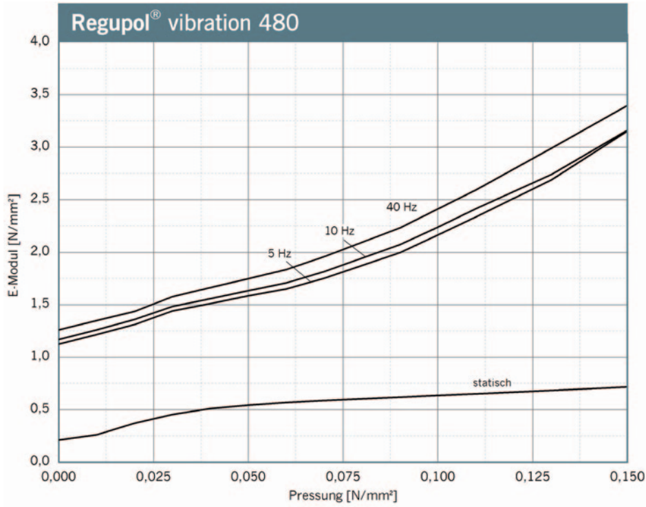
Verlauf des dynamischen E-Moduls bei sinusförmiger Anregung um eine konstante Mittellast, Wegamplitude \pm 0,25 mm. Probenabmessung 300 mm x 300 mm x 45 mm; Statischer E-Modul als Tangentenmodul aus der Federkennlinie. Messung in Anlehnung an DIN 53513.
