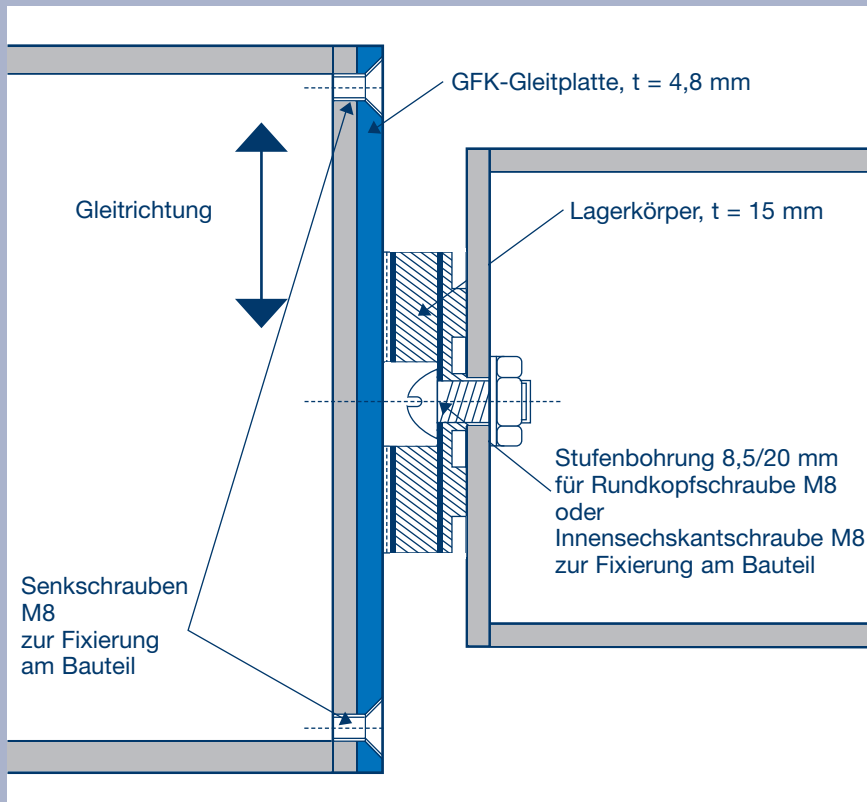
Bild 5: Einbaubeispiel eines Ciparall®-Gleitlagers ST, t = 20 mm, Vertikalfuge zwischen zwei Stahlbauteilen mit Befestigung der einzelnen Lagerkomponenten an den angrenzenden Bauteilen
